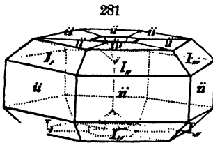
Rutile.
